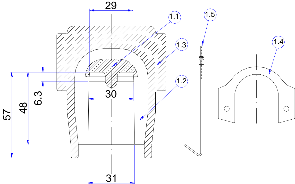
Dimensões em milímetros
